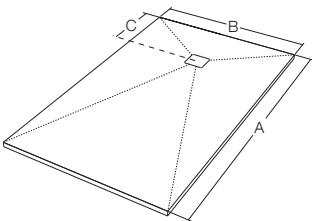
MEDIDAS ESTÁNDAR DISPONIBLES Y DISTANCIA A VÁLVULA STANDARD MEASURES AVAILABLE AND DISTANCE TO VALVE / MESURES STANDARD DISPONIBLES ET DISTANCE À LA VANNE MISURE STANDARD DISPONIBILI E DISTANZA DEL SIFONE / VERFÜGBARE STANDARDGRÖßEN UND ENTFERNUNG ZUM ABLAUF
