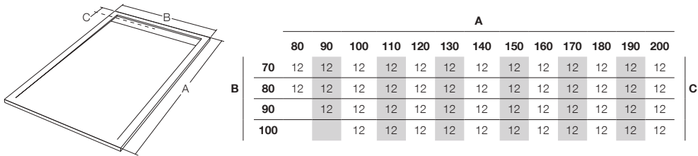
MEDIDAS ESTÁNDAR DISPONIBLES Y DISTANCIA A VÁLVULA STANDARD MEASURES AVAILABLE AND DISTANCE TO VALVE / MESURES STANDARD DISPONIBLES ET DISTANCE À LA VANNE MISURE STANDARD DISPONIBILI E DISTANZA DEL SIFONE / VERFÜGBARE STANDARDGRÖßEN UND ENTFERNUNG ZUM ABLAUF
